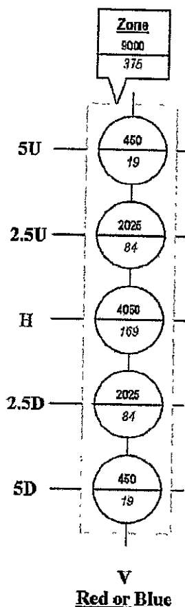
FIGURA 4- REQUISITOS FOTOMÉTRICOS CLASSE 1A e 1S - VERMELHO/AZUL Potência Óptica (Cd-segundos/Minuto) visualizado em Bold (valor superior) Pico de Intensidade Luminosa (Candela) visualizado em Itálico (valor inferior) Fonte: SAE J845 Revised FEB2019, Page 10 of 13.
