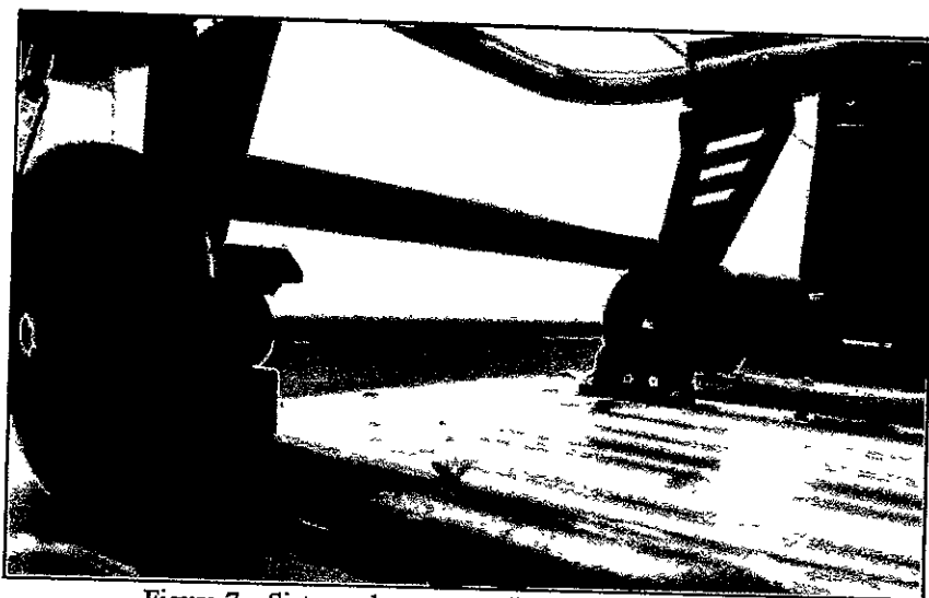
Figura 7 – Sistema de retenção dianteiro após os ensaios
