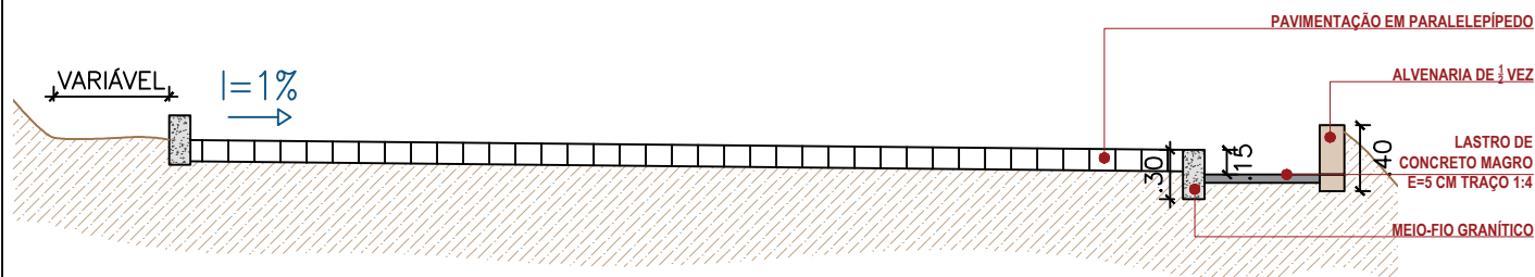
Seção Transversal tipo 01 – ST01 escala → 50
