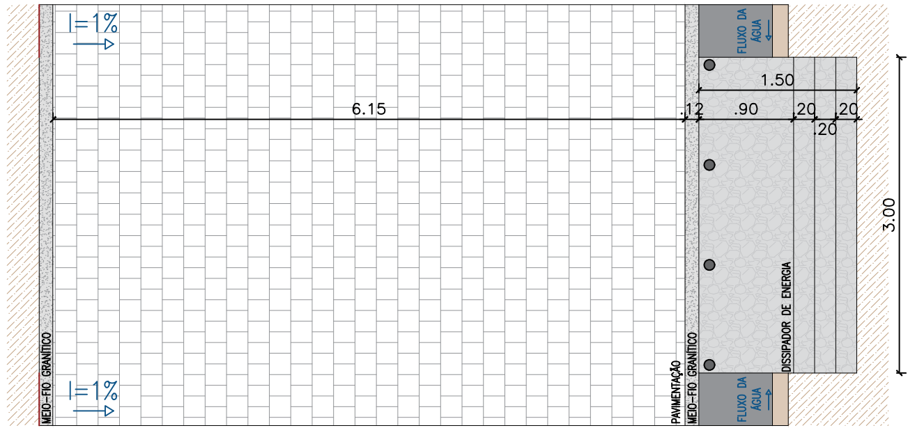
Vista superior – ST02 escala → 50
