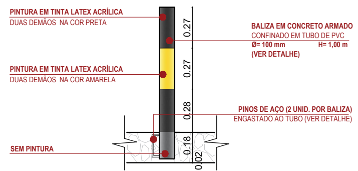
Detalhe de Fixação e pintura das Balizas escala → 1/25
