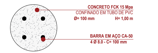
Seção Transversal da Baliza escala → 1/5
