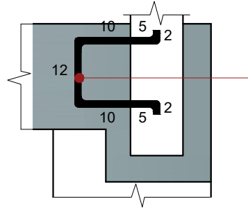
Detalhe – Engaste escala → 1/10
